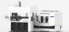
WeStack | Max. Teilgewicht: 15kg Max. Wellenteil: Ø100 L560 Max. Futterteil: Ø140 L100 Autonomiebeispiel Futterteil Ø80 L80 = 448 Stk.
