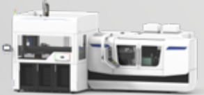
WeStack | Max. Teilgewicht: 15kg Max. Wellenteil: Ø100 L560 Max. Futterteil: Ø260 L100 Autonomiebeispiel Futterteil Ø80 L80 = 448 Stk.
