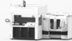
WeStack | Max. Teilgewicht: 15kg Max. Futterteil: Ø260 L100 Autonomiebeispiel Futterteil Ø80 L80 = 448 Stk.
