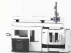
WeFlex mit Dachbeladung Max. Teilgewicht: 15kg Max. Futterteil: Ø260 L100 Autonomiebeispiel Futterteil Ø80 L80 = 200 Stk.
